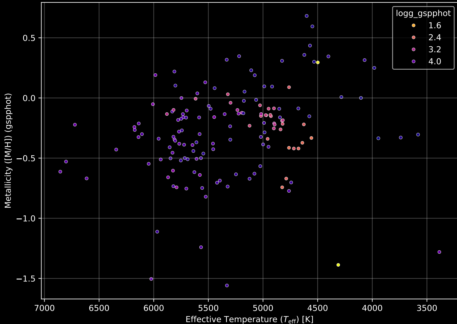
APOGEE DR17 Field: [041+48_MGA] Stellar Population Parameters (n= 150)
